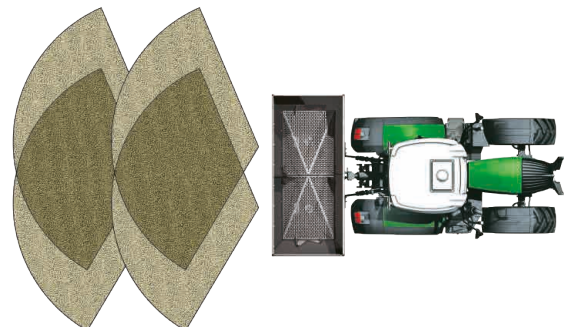
2 vanes per disc
